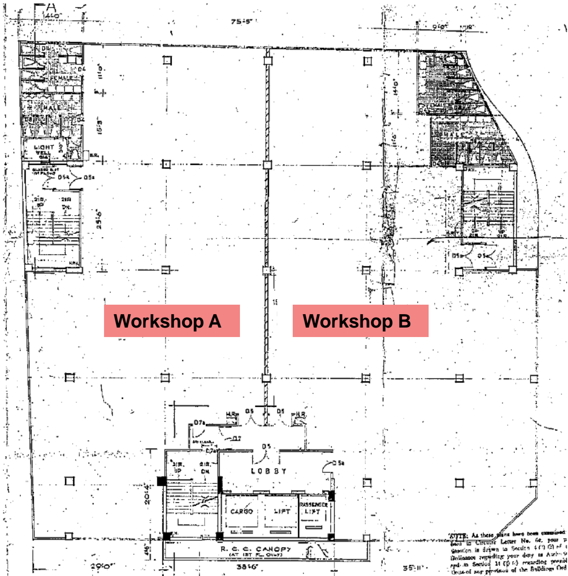
1/F - 3/F 平面圖 Floor Plan
