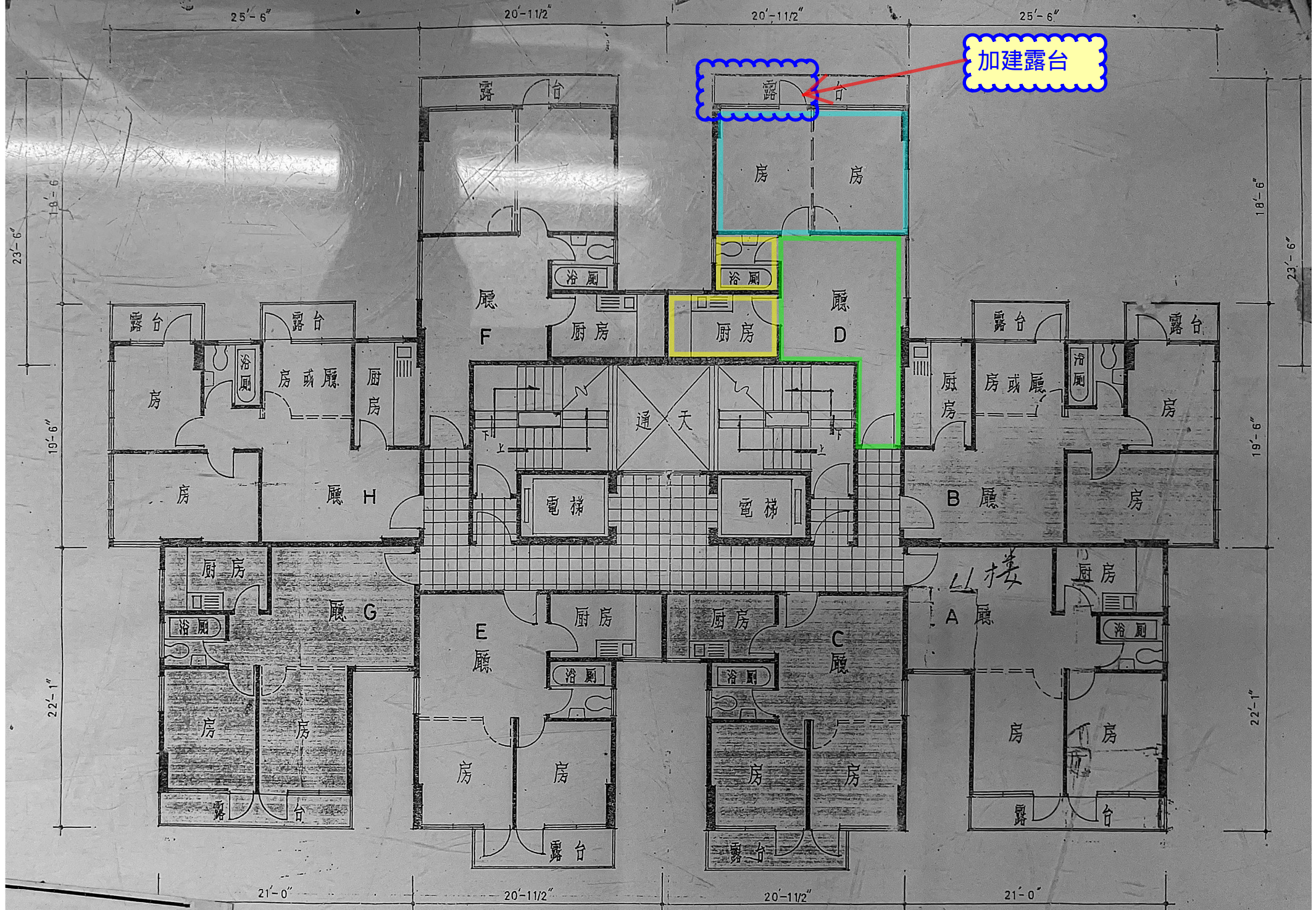
一樓至十二樓平面圖
